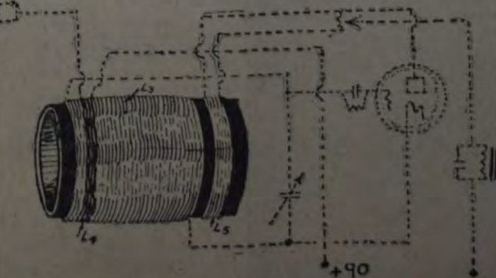
Esquema que muestra cómo se conectan las distintas bobinas del circuito de gran alcance y selectividad cuya explicación iniciamos en el número 7707. La claridad del mismo evita mayores explicaciones.
